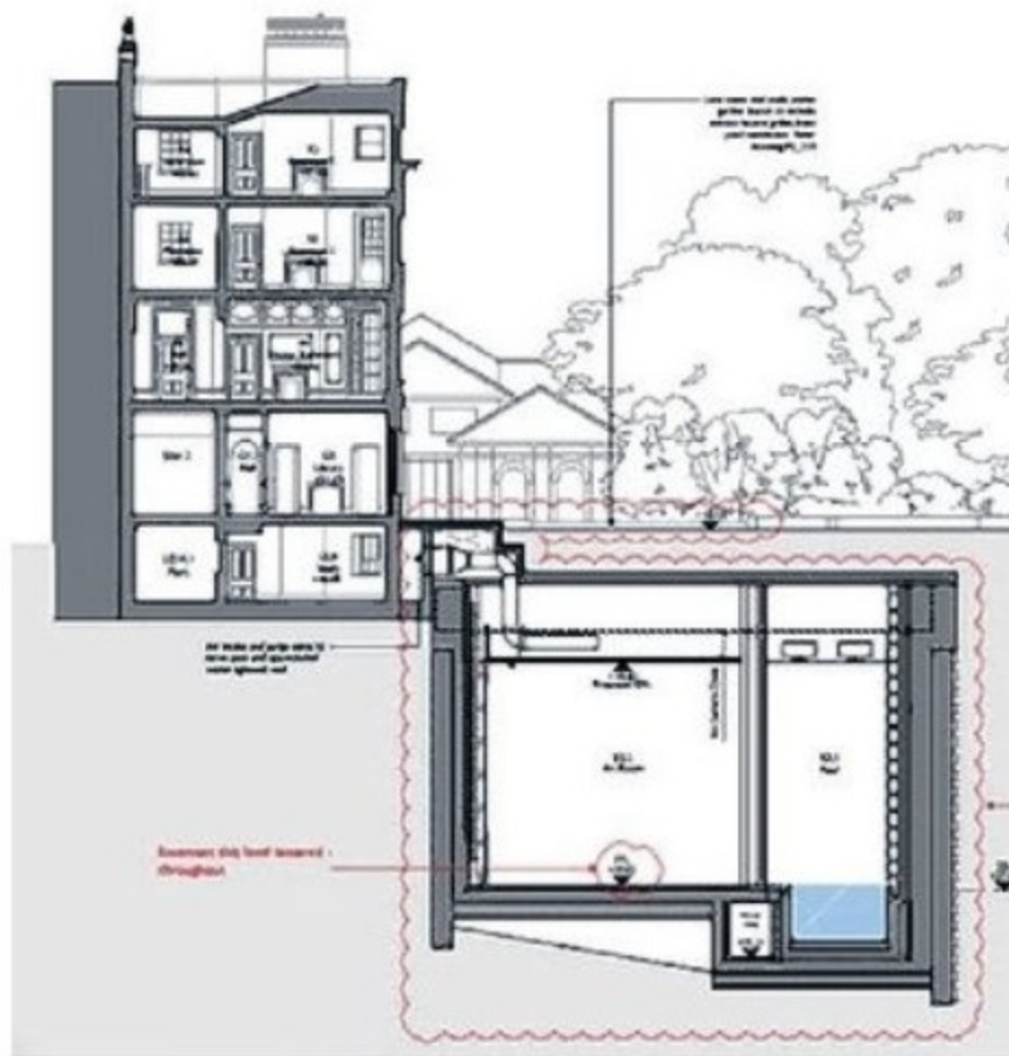
Dwarsdoorsnede van de villa met souterrain met zwembad.
